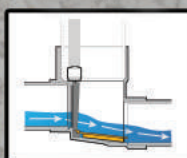
Débit Normale
